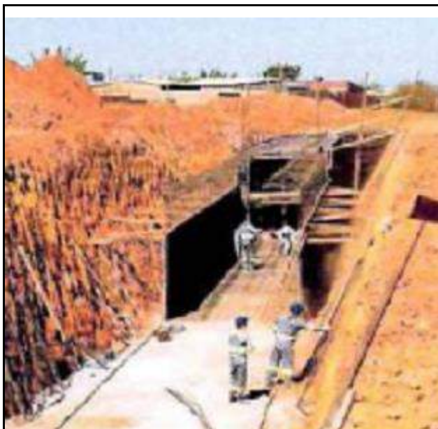
Foto 3: Tunnel liner de travessia sob a rede 14 e galeria celular de concreto
