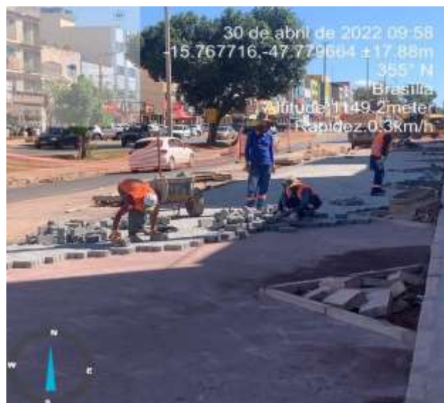
Assentamento de blocos de concreto intertravados
