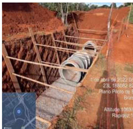
Assentamento de tubos de concreto
