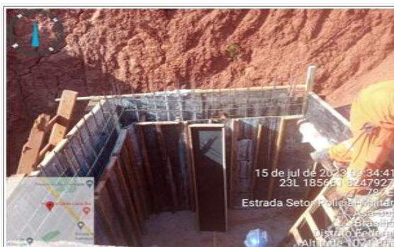
Execução de poço de visita.
